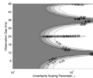
(d) P_{FA} = 0.1
