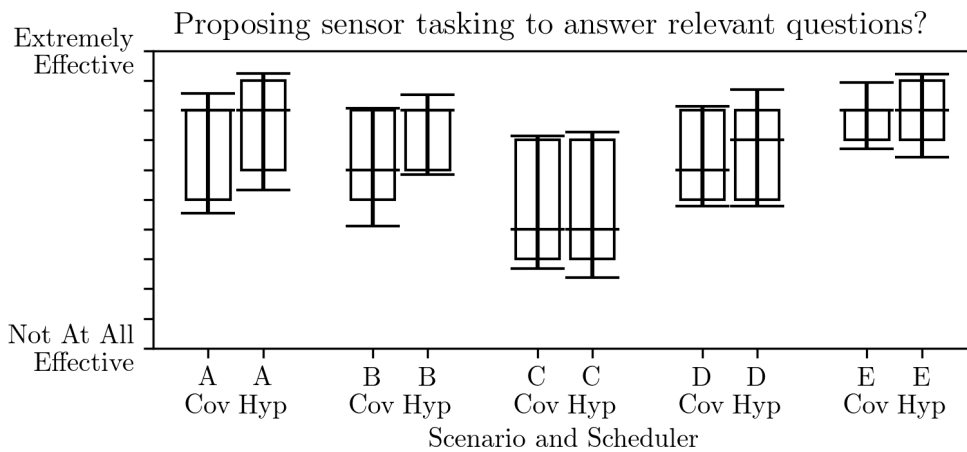
(b) Prompt 2
