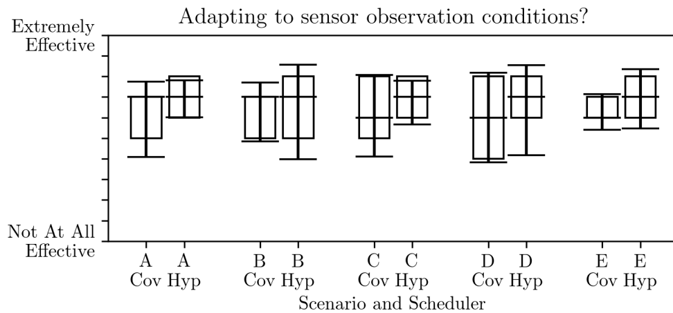
(b) Prompt 8
